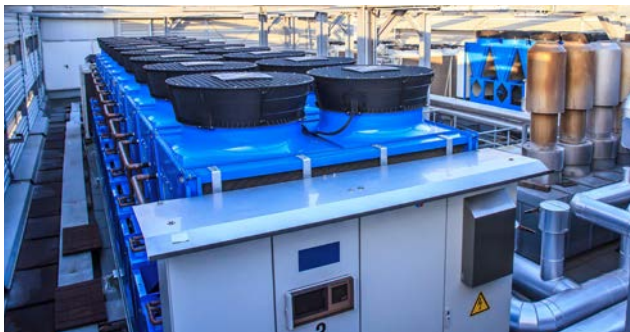
Außenkühlung und zentrale Zu- und Abluftversorgung
